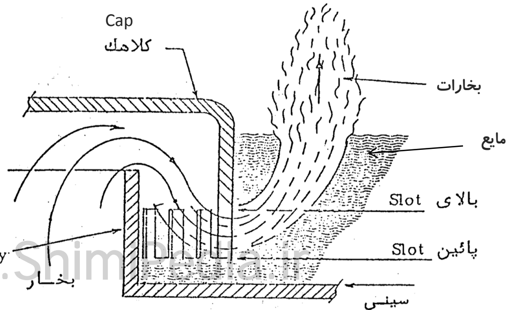
اجزای یک سینی با کلاهک حبابی
